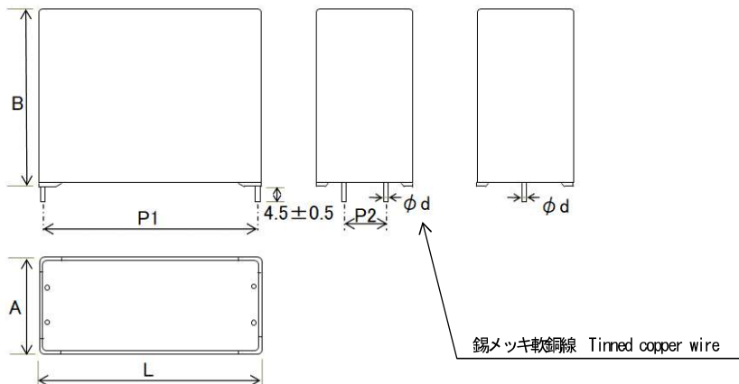
■ 外形図 Component outline
