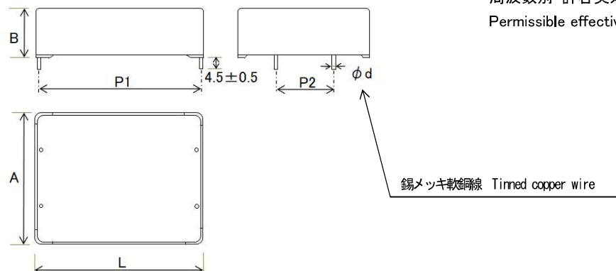
■ 外形図 Component outline
